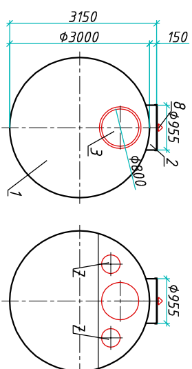
Вид сверху
