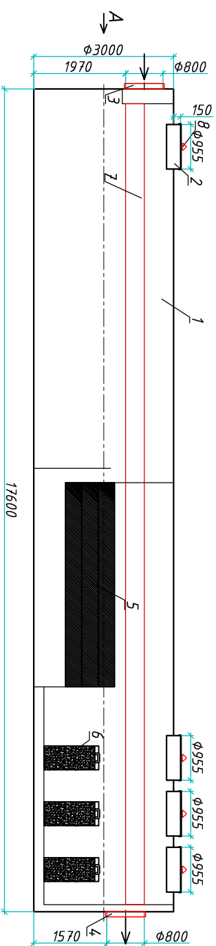
Разрез 1-1
